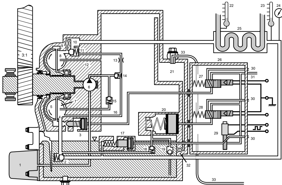
Diagrama hidráulico
